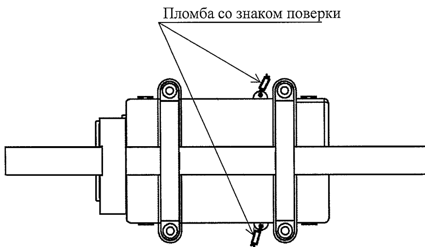
Рисунок 5 – Схема пломбировки от несанкционированного доступа, обозначение места нанесения знака поверки ДИЭ
