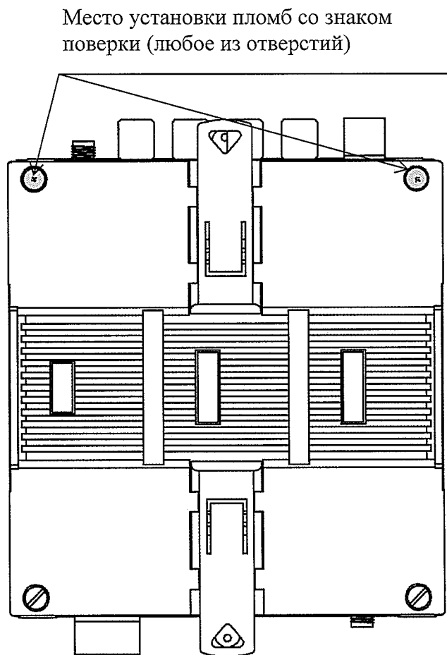
Рисунок 4 – Схема пломбировки от несанкционированного доступа, обозначение места нанесения знака поверки ББ
