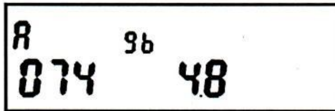
Рисунок 5 – Пример индикации параметров связи по интерфейсу RS-485 (адрес в магистральной RS-485 – 074, скорость обмена 4,8 кБод, режим 9-ти битной передачи данных)
